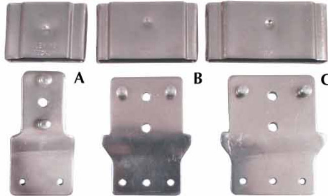
All Metal Blevins Buckles A. No. 11120 2" B. No. 11121 2 1/2" C. No. 11122 3"
